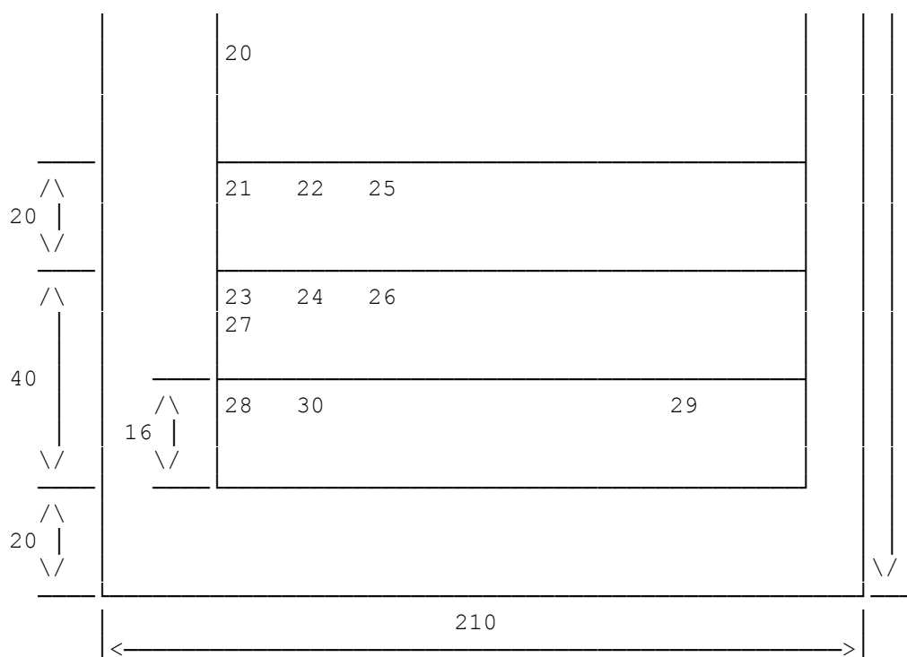
Рисунок А.1. Расположение реквизитов и границы зон на формате А4 углового бланка
