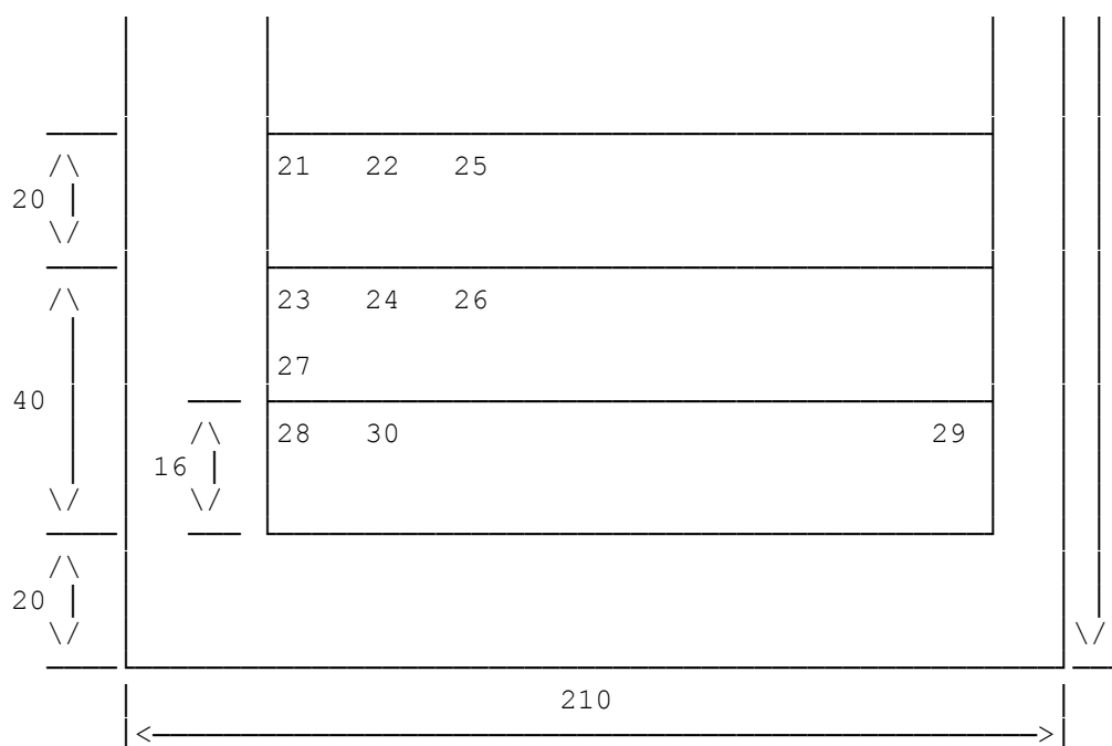
Рисунок А.2. Расположение реквизитов и границы зон на формате А4 продольного бланка
